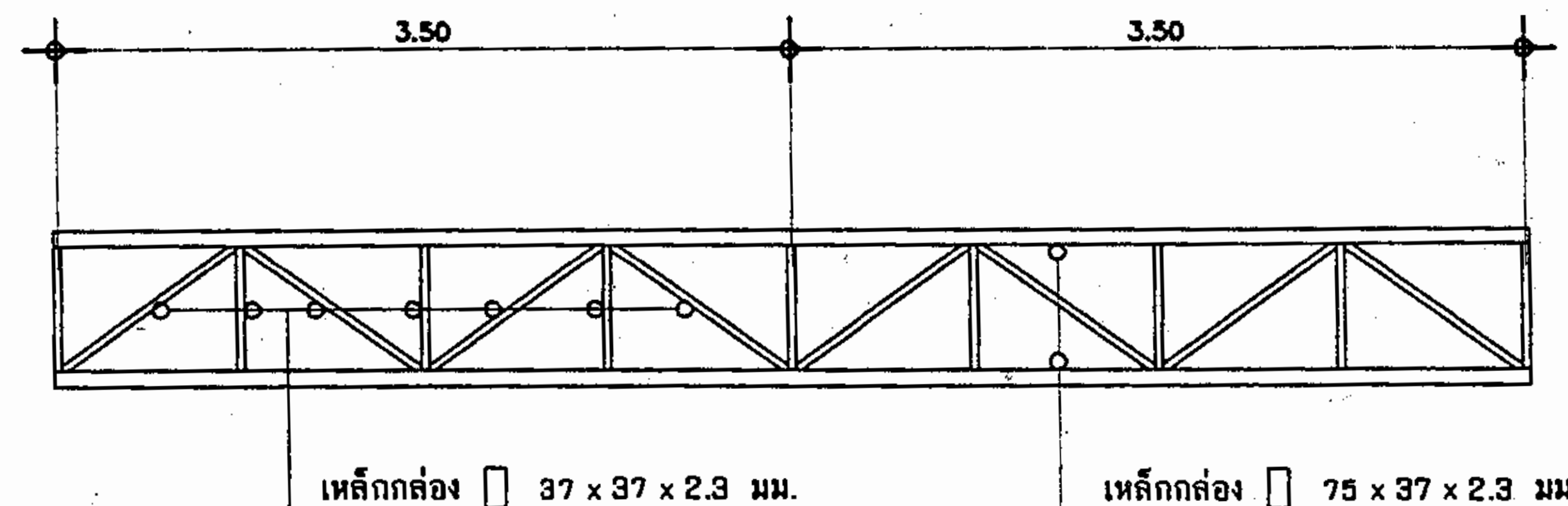
ขยาย TRUSS 1 1 : 50
