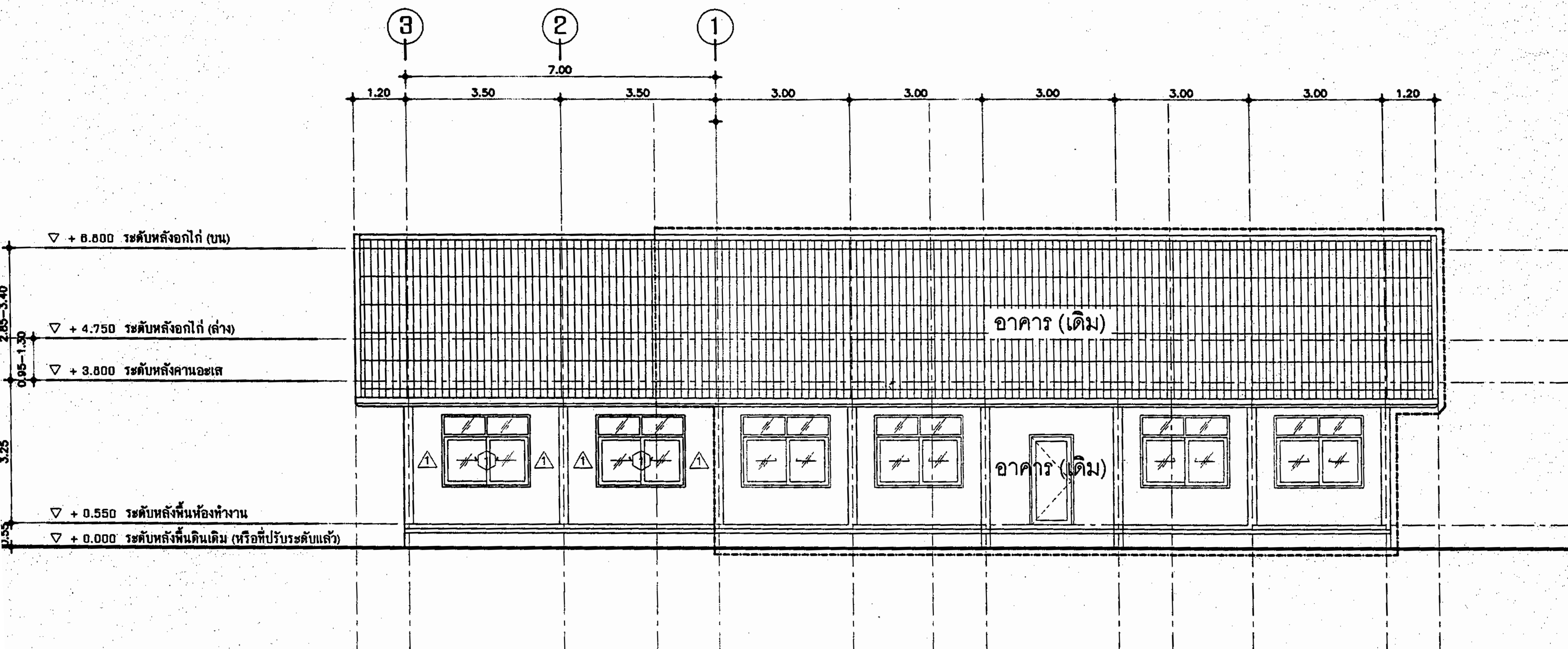
รูปตัดด้าน C 1 : 100
