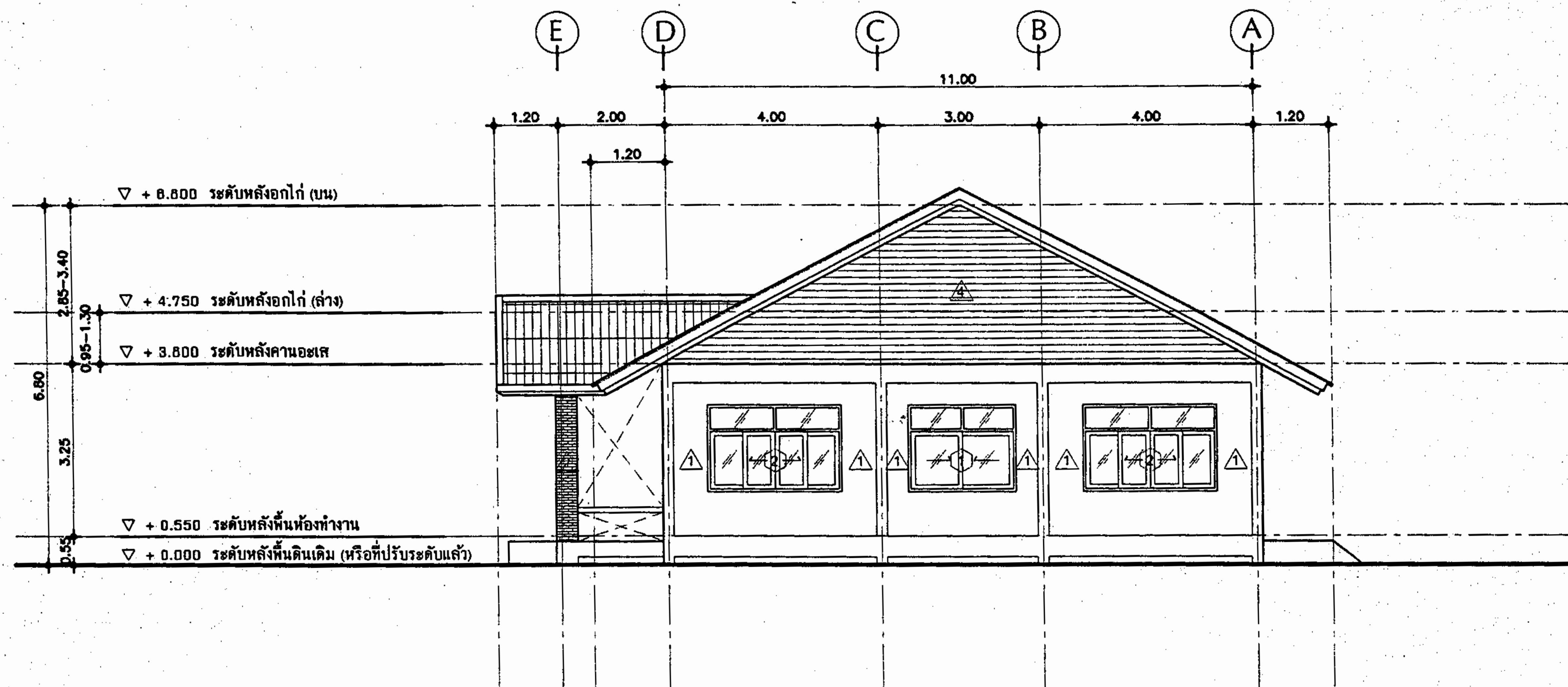
รูปตัดด้าน B 1 : 100
